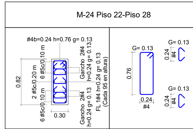
DETALLE SOBRE ANCHO EN MURO M-24 Escala 1 : 25
