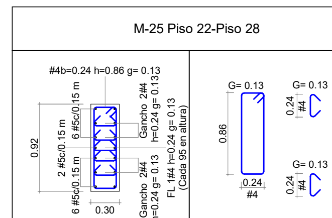
DETALLE SOBRE ANCHO EN MURO M-25 Escala 1 : 25
