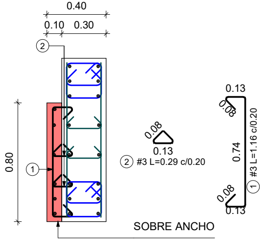
DETALLE SOBRE ANCHO EN MURO M-26 Escala 1 : 25
